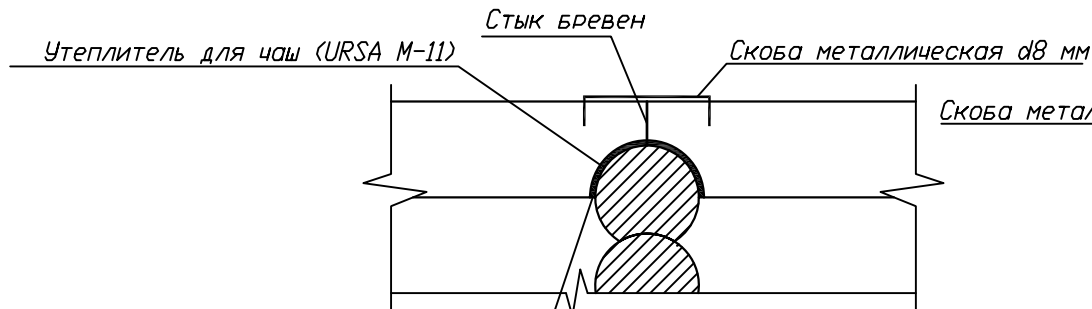
Схема сопряжения бревен по длине
