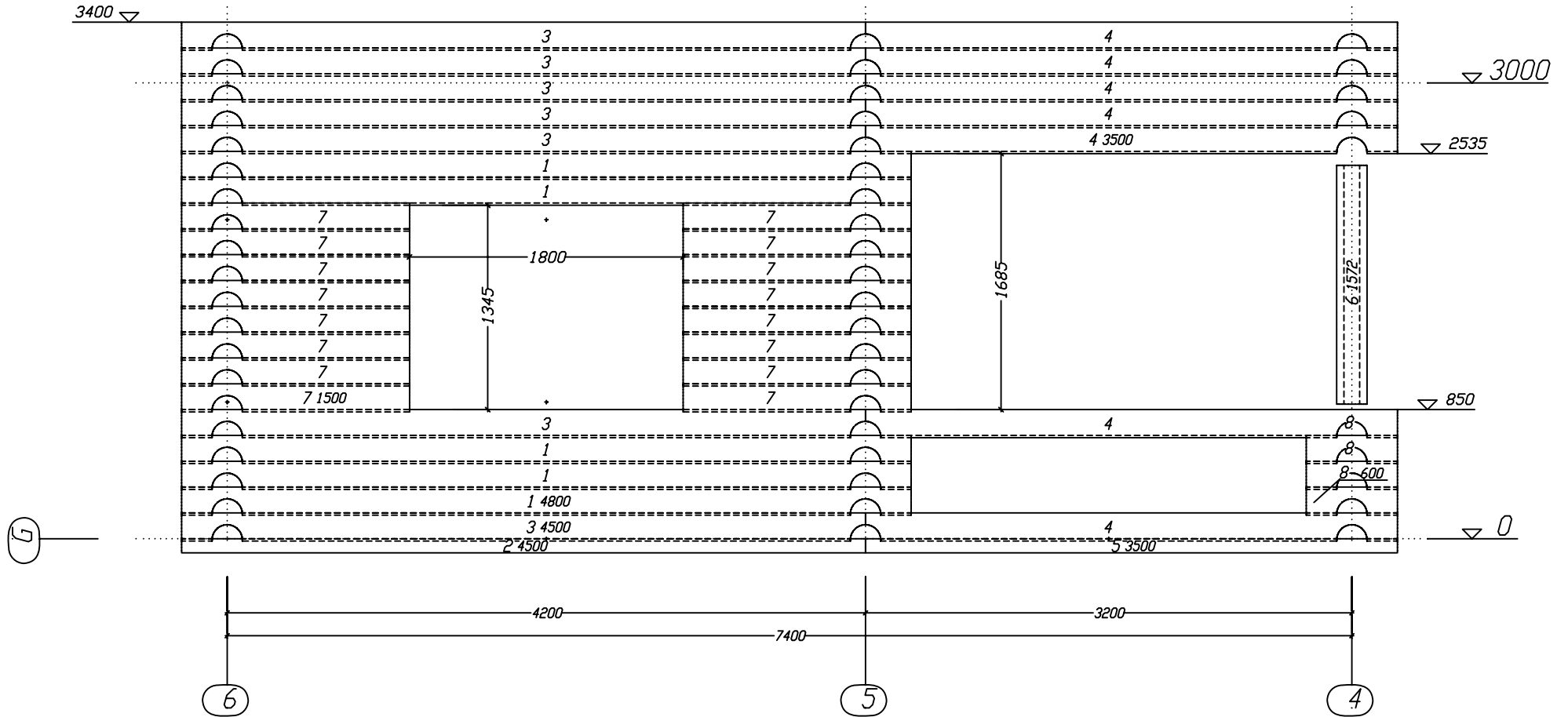
СПЕЦИФИКАЦИЯ СТЕНЫ 16
