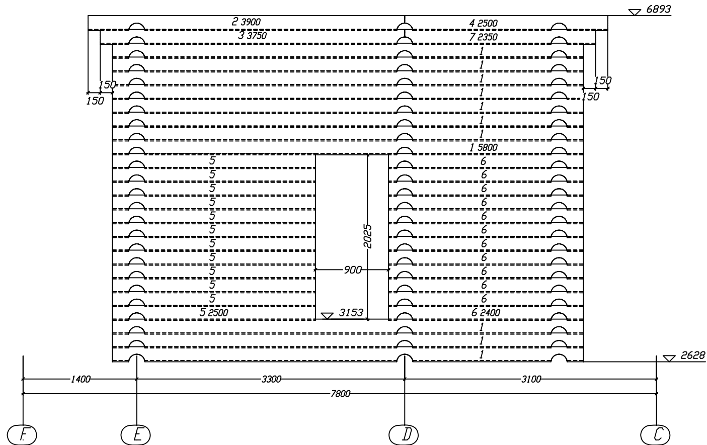
СПЕЦИФИКАЦИЯ СТЕНЫ 18
