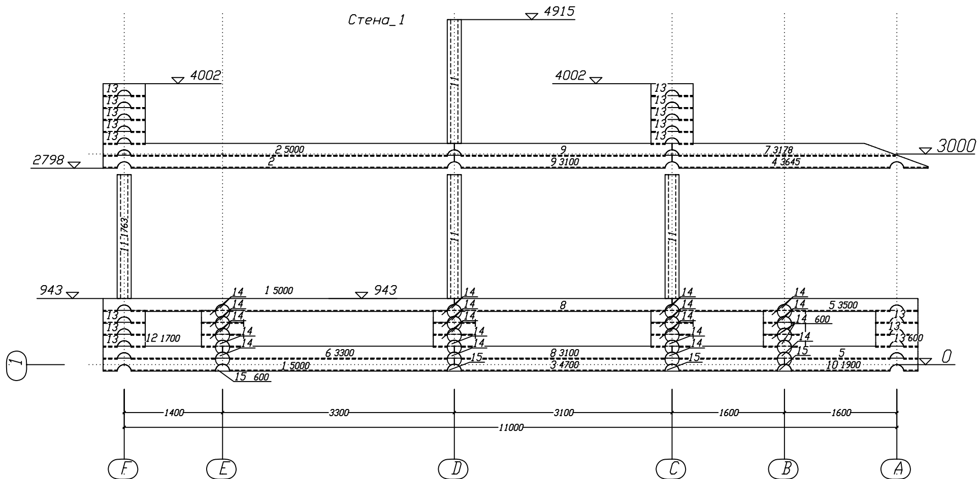
СПЕЦИФИКАЦИЯ СТЕНЫ 1
