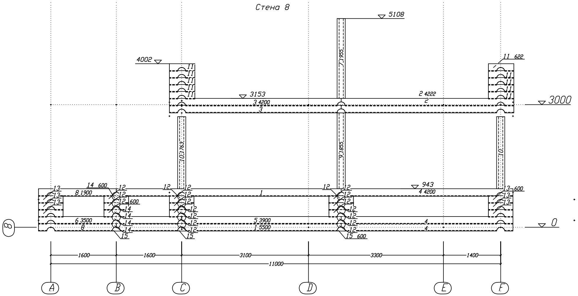
СПЕЦИФИКАЦИЯ СТЕНЫ 8
