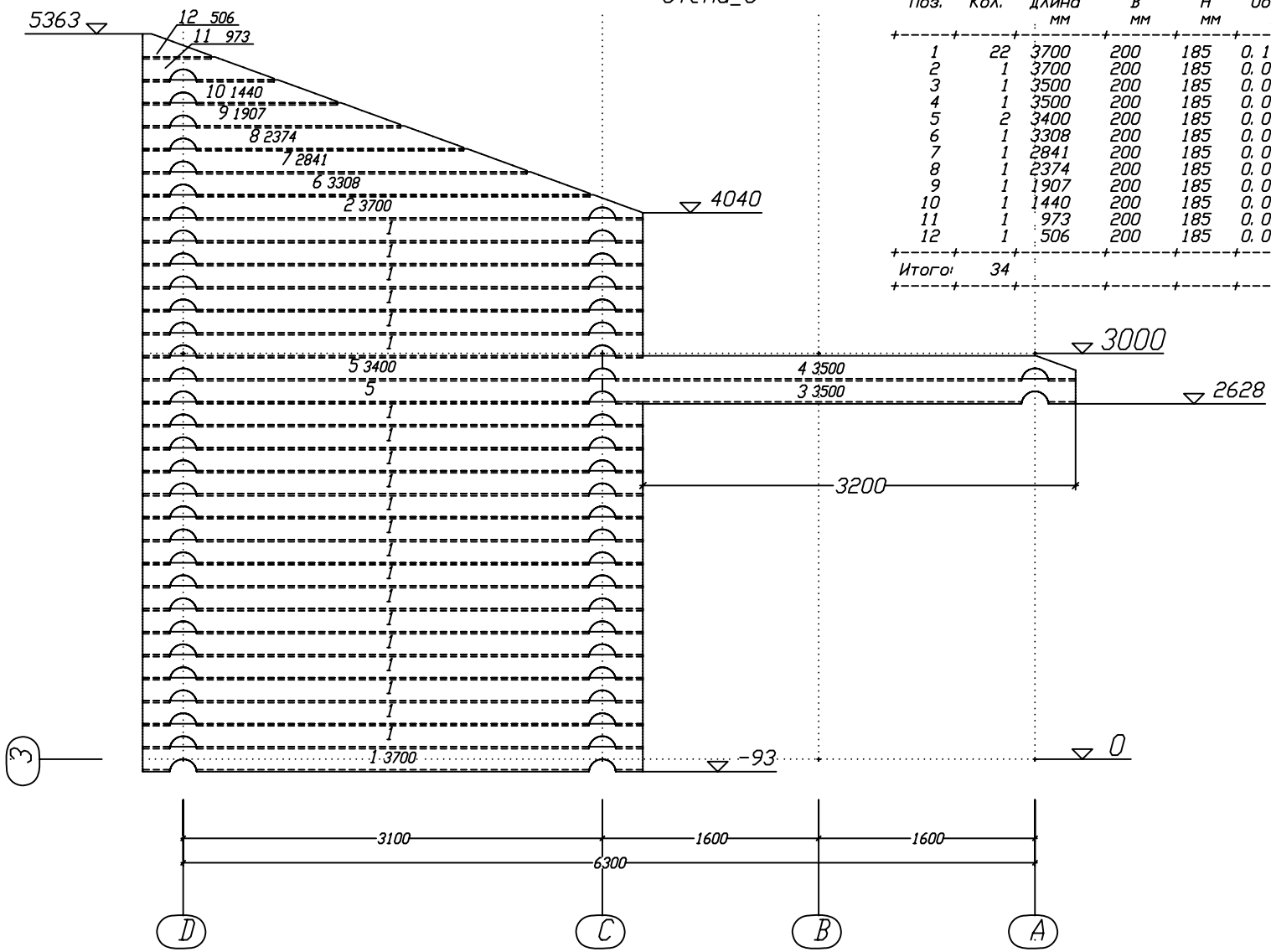
СПЕЦИФИКАЦИЯ СТЕНЫ 3
