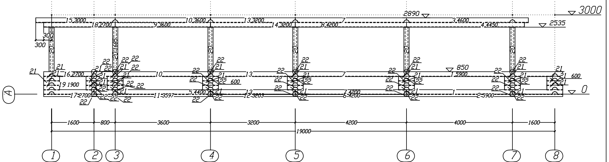
СПЕЦИФИКАЦИЯ СТЕНЫ 9
