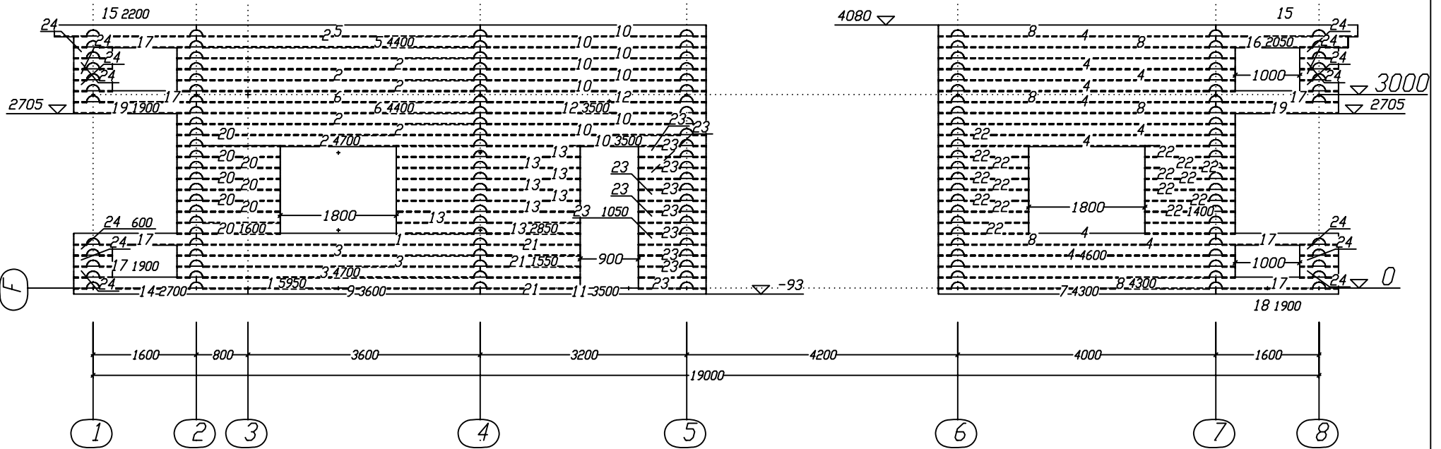
СПЕЦИФИКАЦИЯ СТЕНЫ 15
