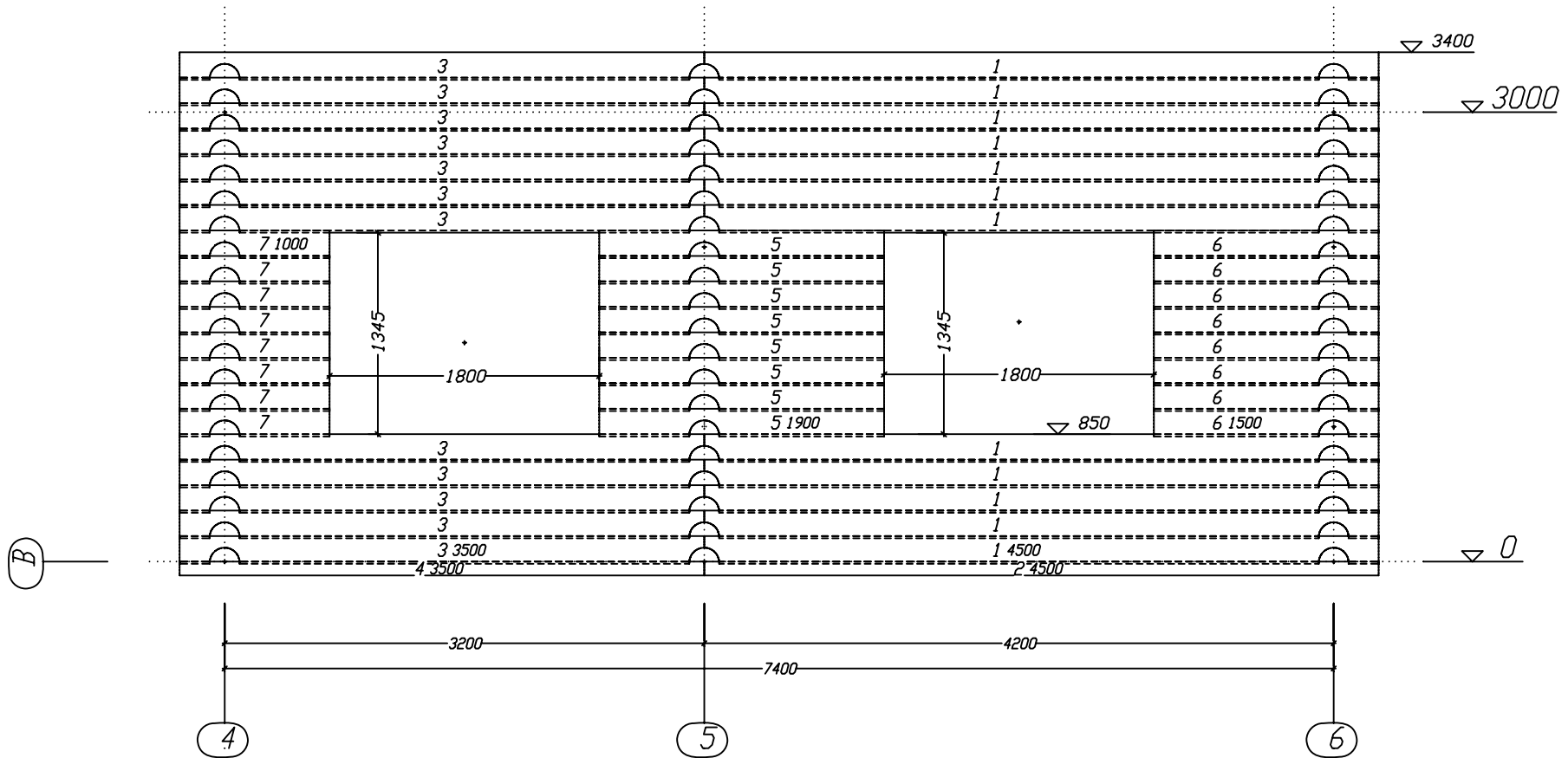
СПЕЦИФИКАЦИЯ СТЕНЫ 10
